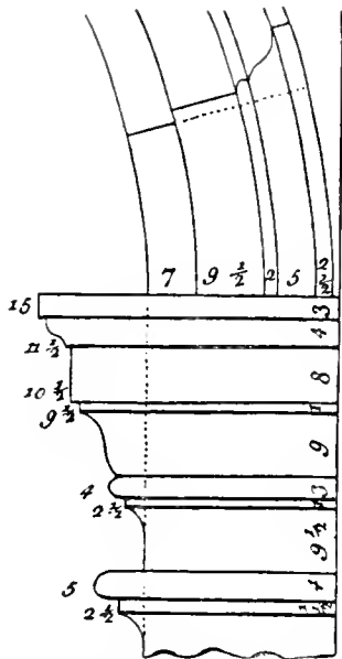
No. 221.—DORIC IMPOST AND ARCHIVOLT MOULDINGS.
